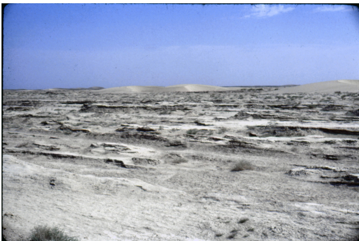
Шакли 14.8: Фарсоиши боднои кавӣ 120 рӯза боис шуд, ки тарсбот энгиқол ва интиқол дода шавад
