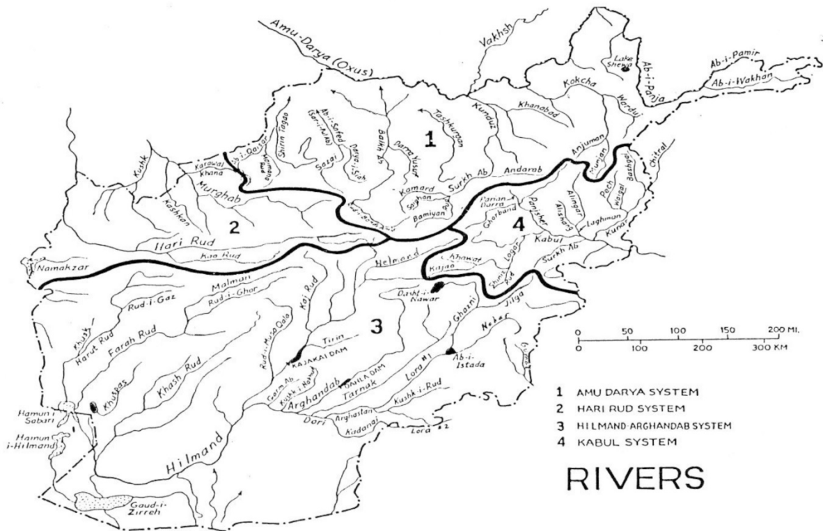
Шакли 14.1: Дар нақшаи оби Афғонистон навъҳои дарёи Нилманд дар шумораи савуми Ҳарируд – Марғоб дар шумораи дувум нишон дода шудааст.
