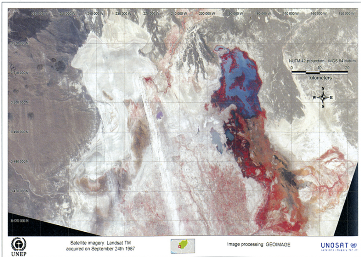
Ш акли 14.6 Б: Тасвири қамари маснуъии навзаи Сиистон дар соли 1987 мелодӣ .
