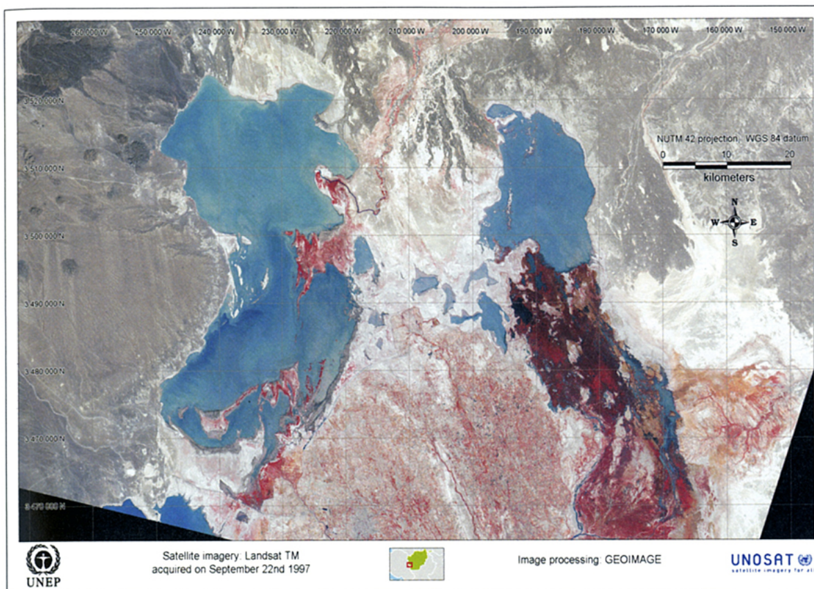
Ш акли 14.6 В: Тасвири қамари маснуъии навзаи Сиистон дар соли 1998 мелодї .
