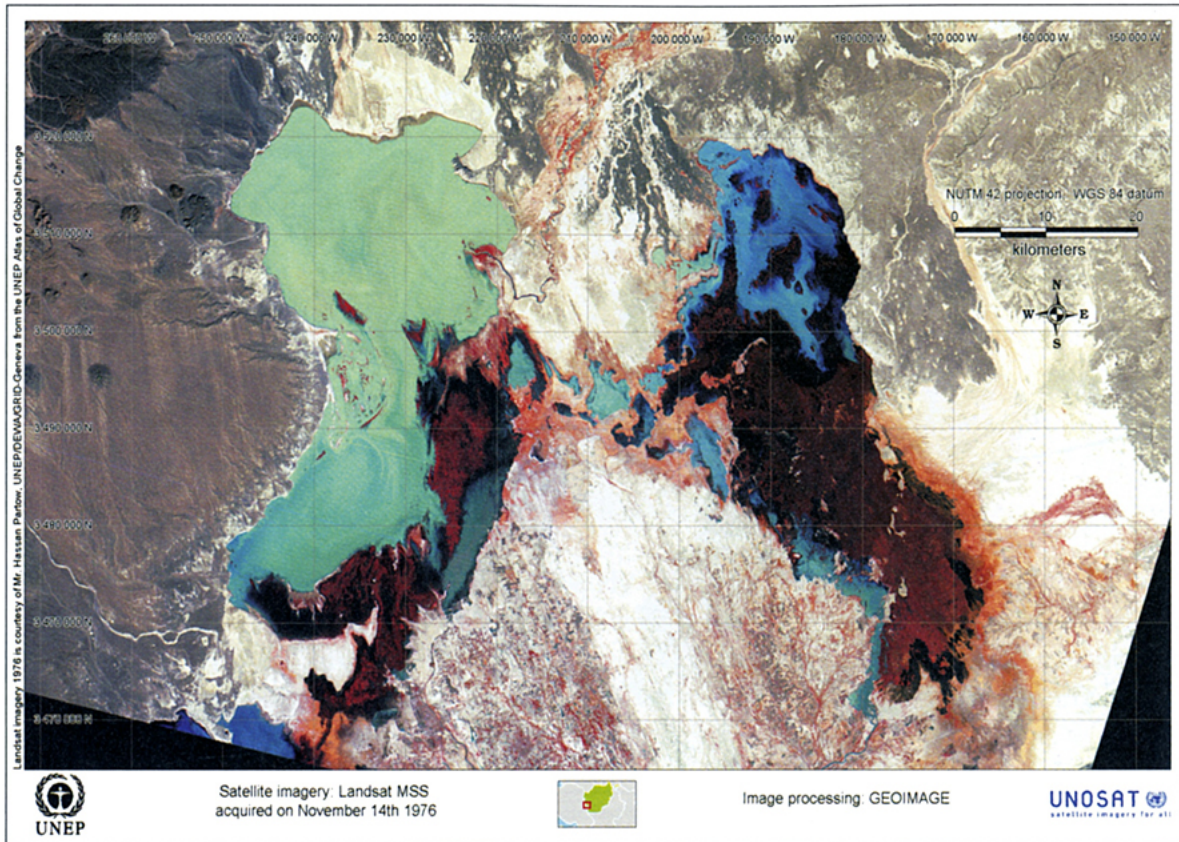
Ш акли 14.6 А: Тасвири қамари маснуъии ҷавзаи Сиистон дар соли 1976 мелодӣ .
