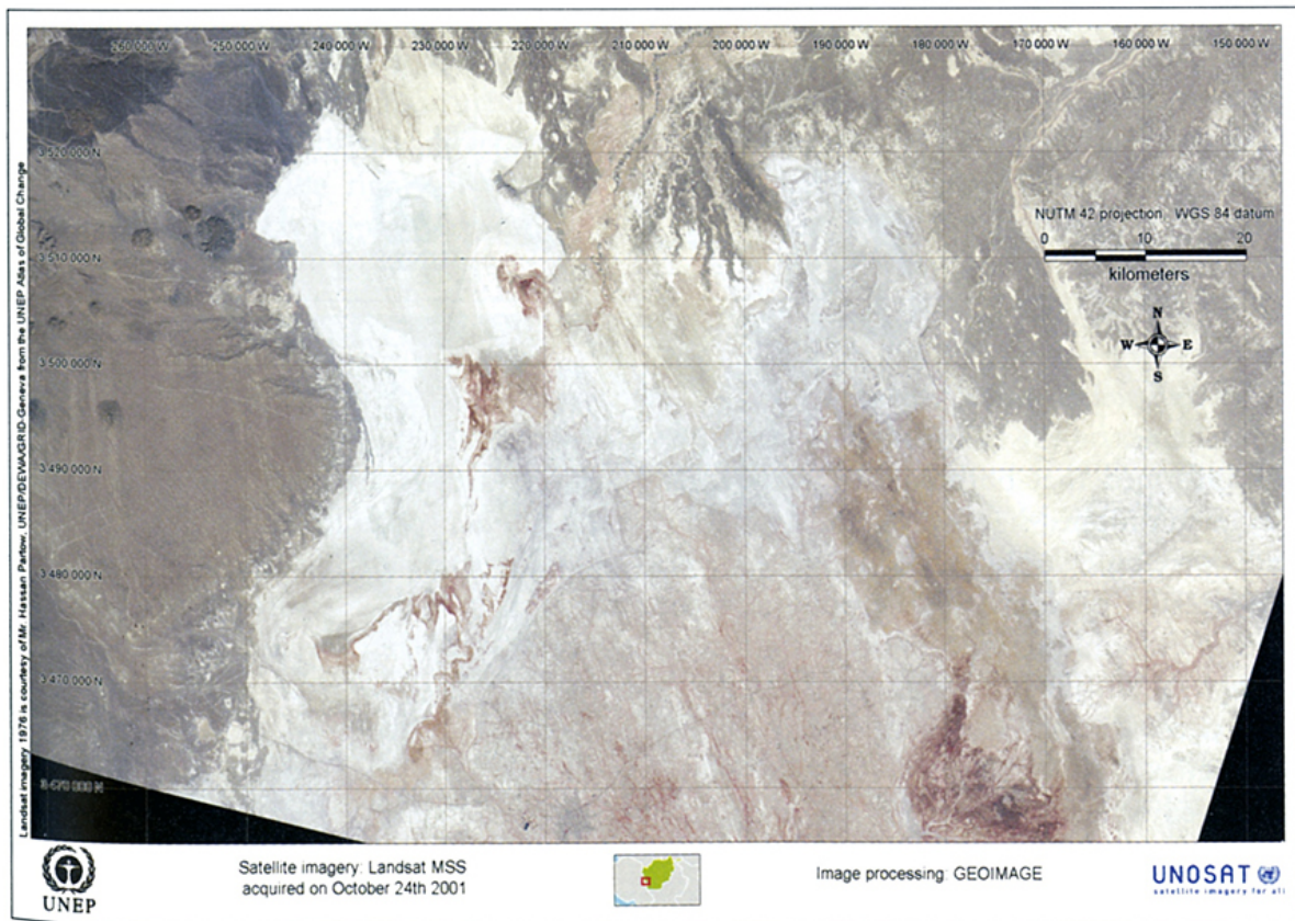
Ш акли 14.6 Г 2: Тасвири қамари маснуъии навзаи Сиистон дар соли 2001 мелодӣ .
