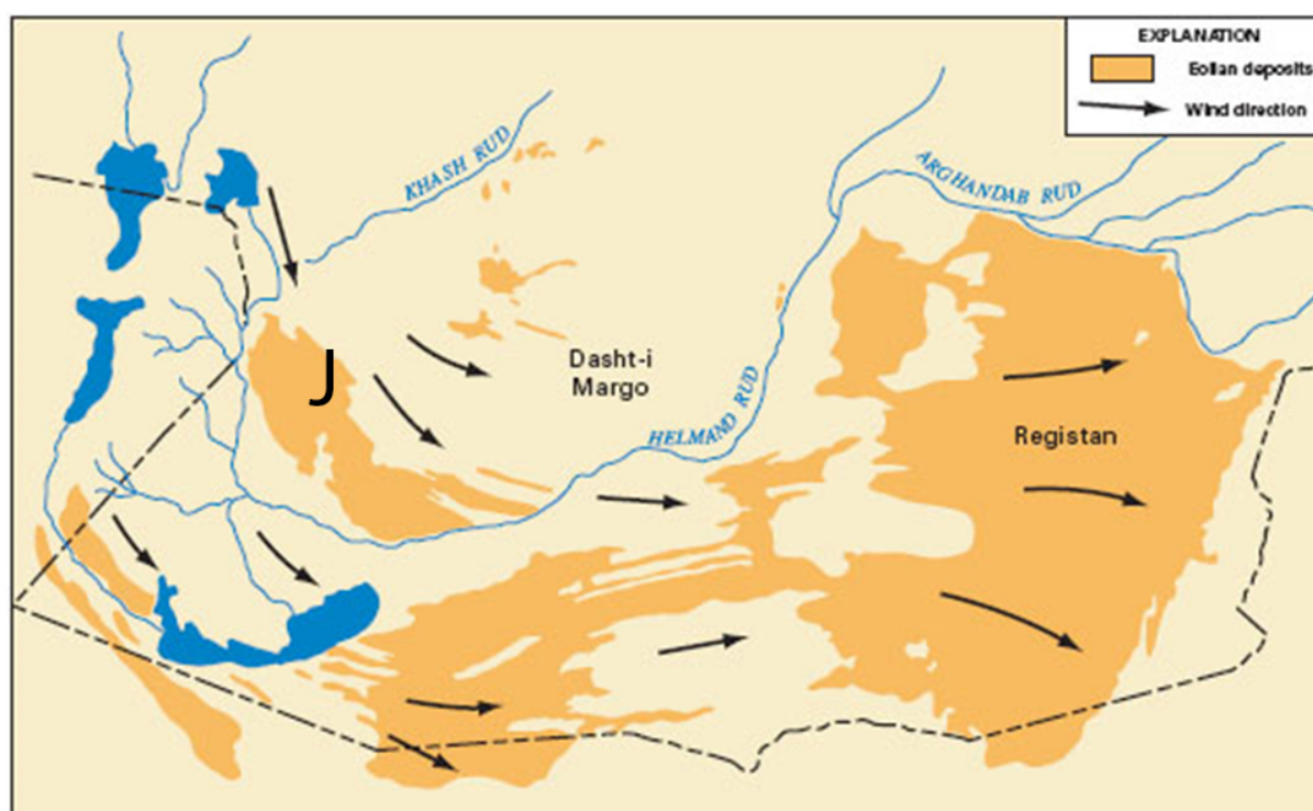
Шакли 14.10: Нақшаи бод шудани рег дар фуруфтагии Сиистон масири самти бодро ва дар теппаю наракати регро нишон мединад.
