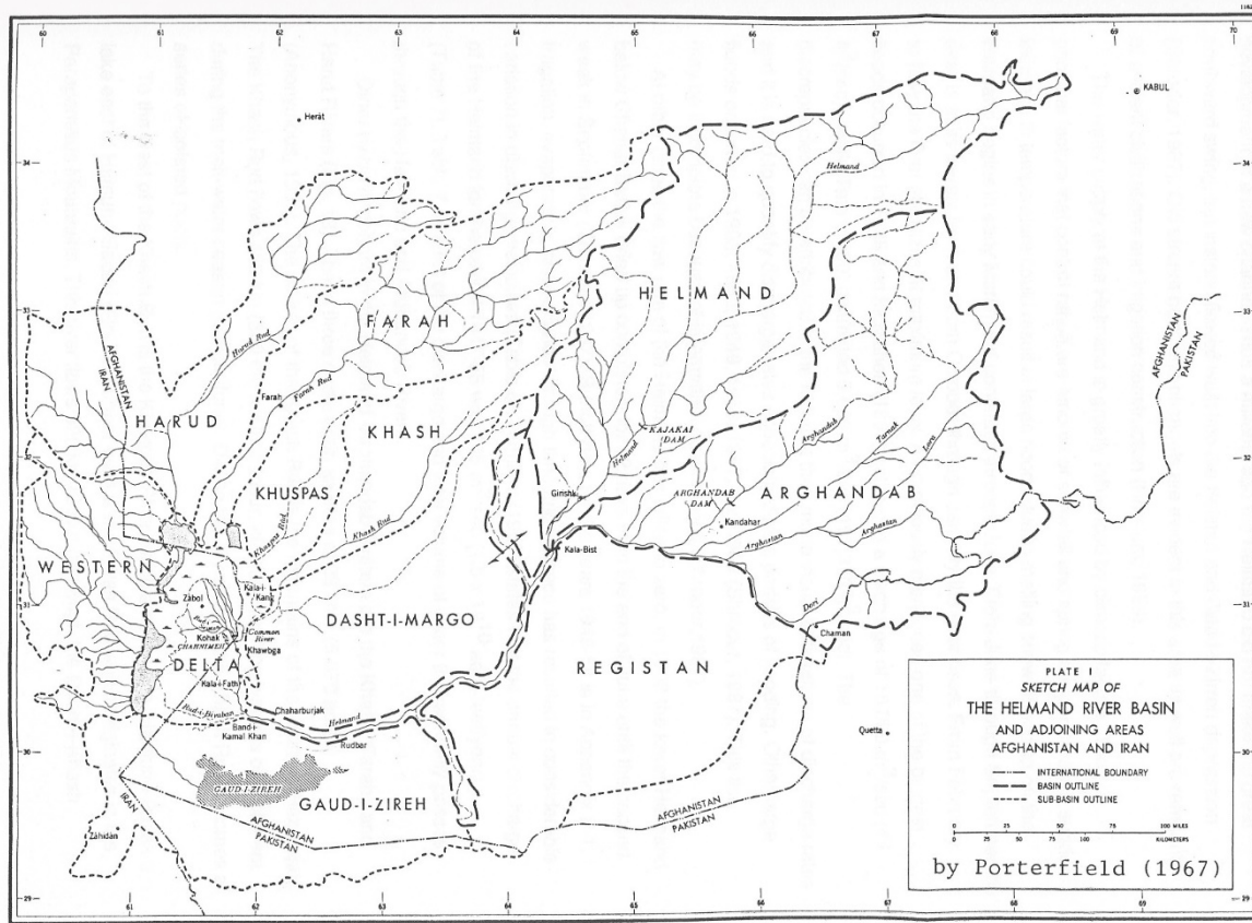
Ш акли 14.2: Лузъиёти навзай дарёи Ўилманд.
