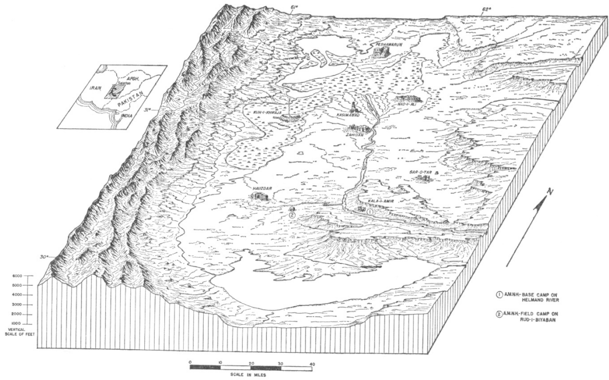
Ш акли 14.4: Манзара ба шакли кортун расм шудааст. Дар ин расм дотҳои дарёи Нилманд расм шудааст ва дар он ишон дода шудааст, ки чӣ гуна ҷараёни оби пеш аз ин ки ба Гудзара, ки як соҳаи фурурафта аст ва дар пешравиҳои ҷараёни об воқеъ аст, бирасад ба самти муқолифи ақрабаки соат наракат мекунад.
