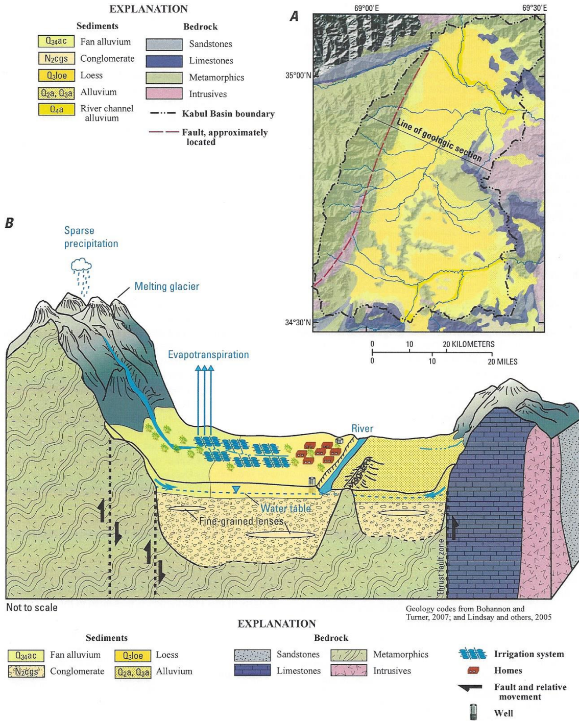
Шакли 4-12: Дар болои нақша ва дар қисмати пойини расми ҳавзаи зерзаминии Кобул ба сатҳи оби зери шахр памп мешавад, дида мешавад, бори дигар аз ҷойе, ки дарё ё ҷаҳил аст, об ба тарафи пойин аз тариқи соҳаи Сурубӣ нуфуз мекунад ва эҳё мешавад.
