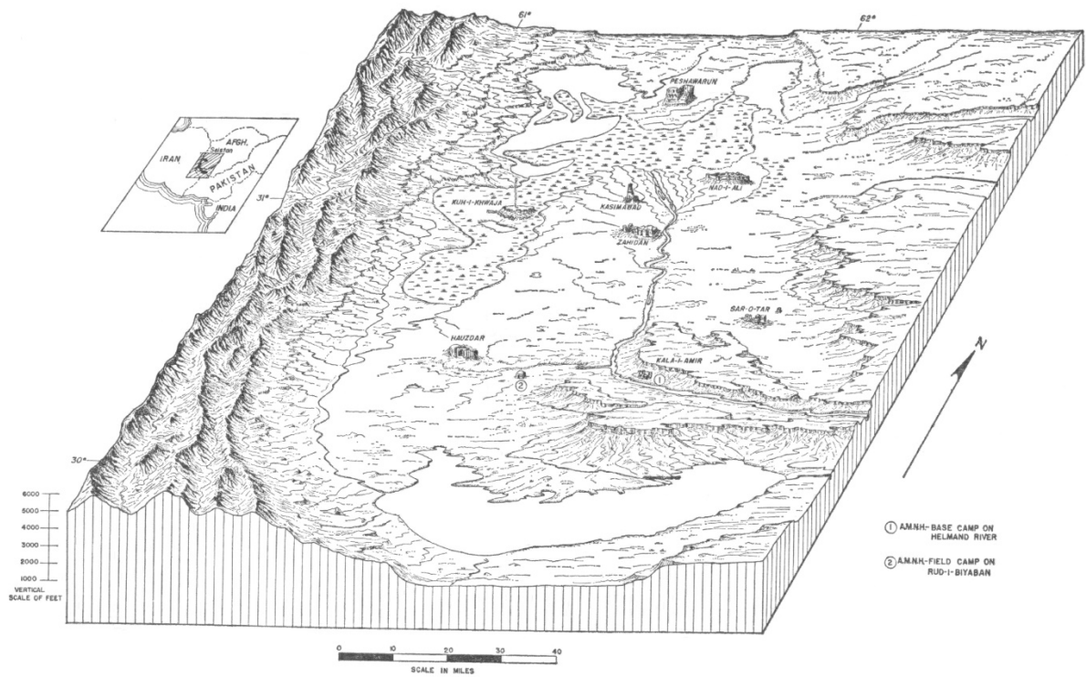
Шакли 4-8 Б: Тарсими соҳаи Дилтои Хелманд дар охири ҳавзаи Сиистон, ҷойе, ки ҷаҳил хушк шудааст. Ҷаҳили Ҳасаки Гавдзарра як соҳаи густурдаи сафед дар қисмати ахирии маркази тасвир нишон дода шудааст.
