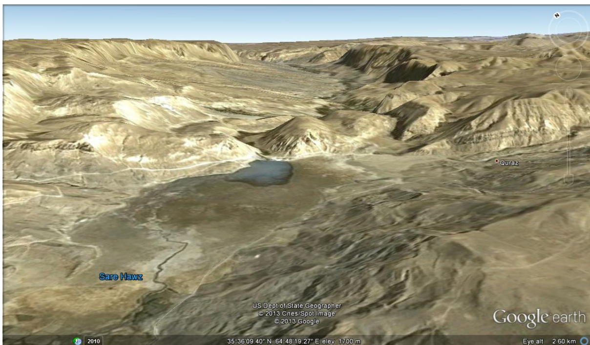
Шакли 4-9: Тасвири камари маснуъии соҳаи sari howz дар шимоли шарқ ҷойе, ки шикастагӣ боис шуда, ки ахҷорро боло оварда дарёро сад сохтааст.
