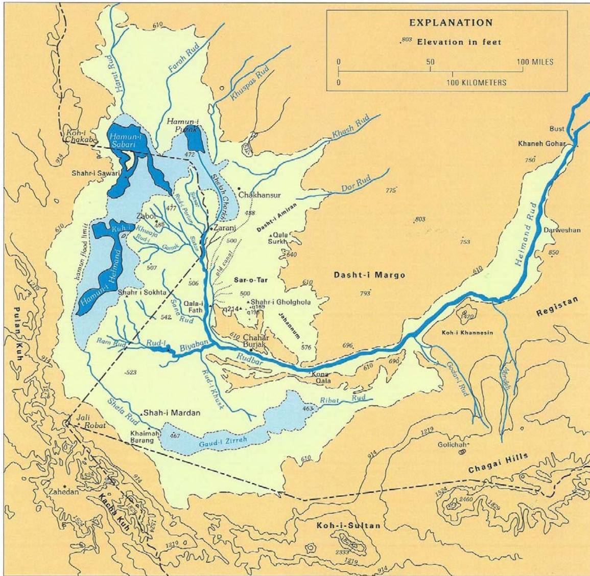
Шакли 4-7 Б: Нақшаи феълии дарёи Ҳелманд, чойе, ки барфи Ҳиндикӯш об мешавад ва билохира ба чаҳили Ҳомун, ки мавсимӣ аст, мерезад.
