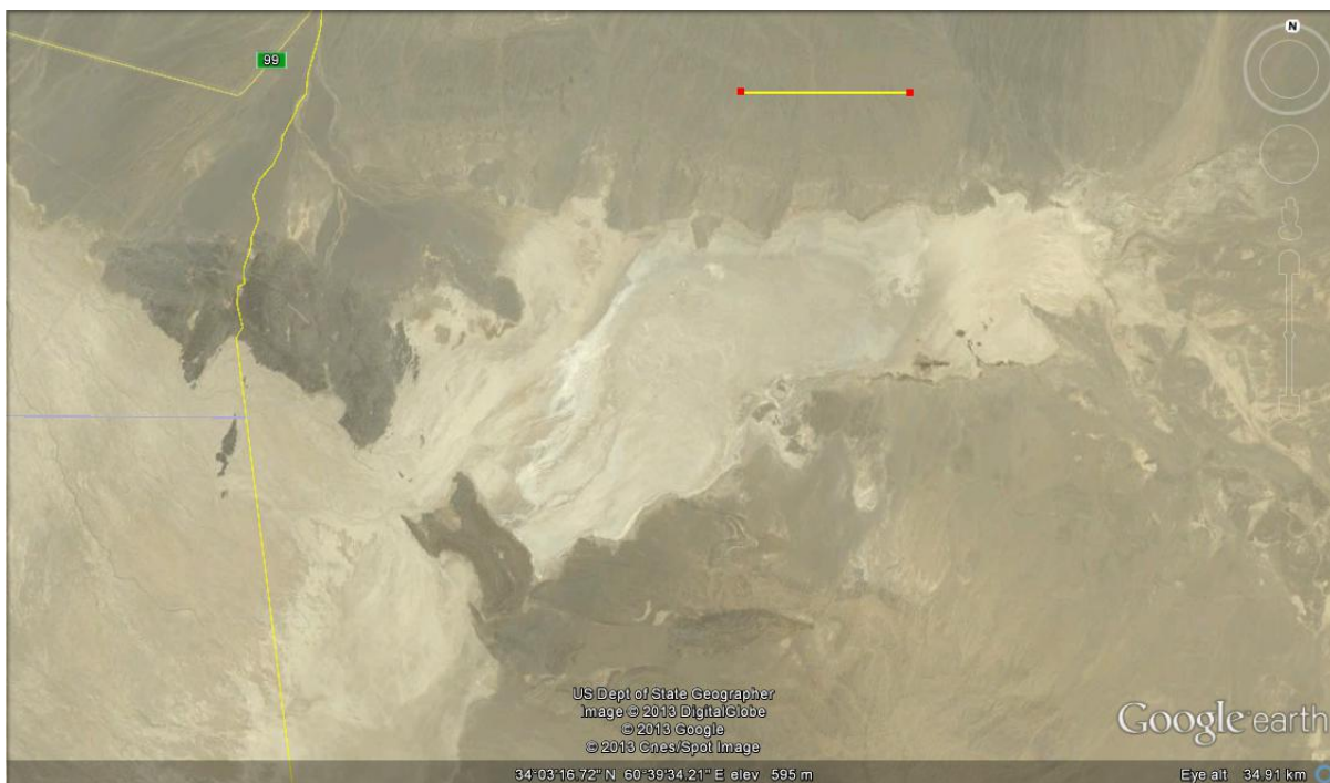
Шакли 4-5 А: Намаксори Хирот дар сарҳади Эрон чаҳили намаки хушк аст, ки милиунҳо сол қабл тавассути вурӯ рафтани шикастагӣ- чойе, ки куҳҳои сангӣ дар атрофи он шикаст ва ба тарафи пойин фуру рафт. Миқёс дар бахши васатӣ аққалан 5km тул дорад. Хатти зарде, ки ба боло ва пойин имтидод ёфта дар чапи он сарҳади байналмилалиро бо Эрон нишон медиҳад.
