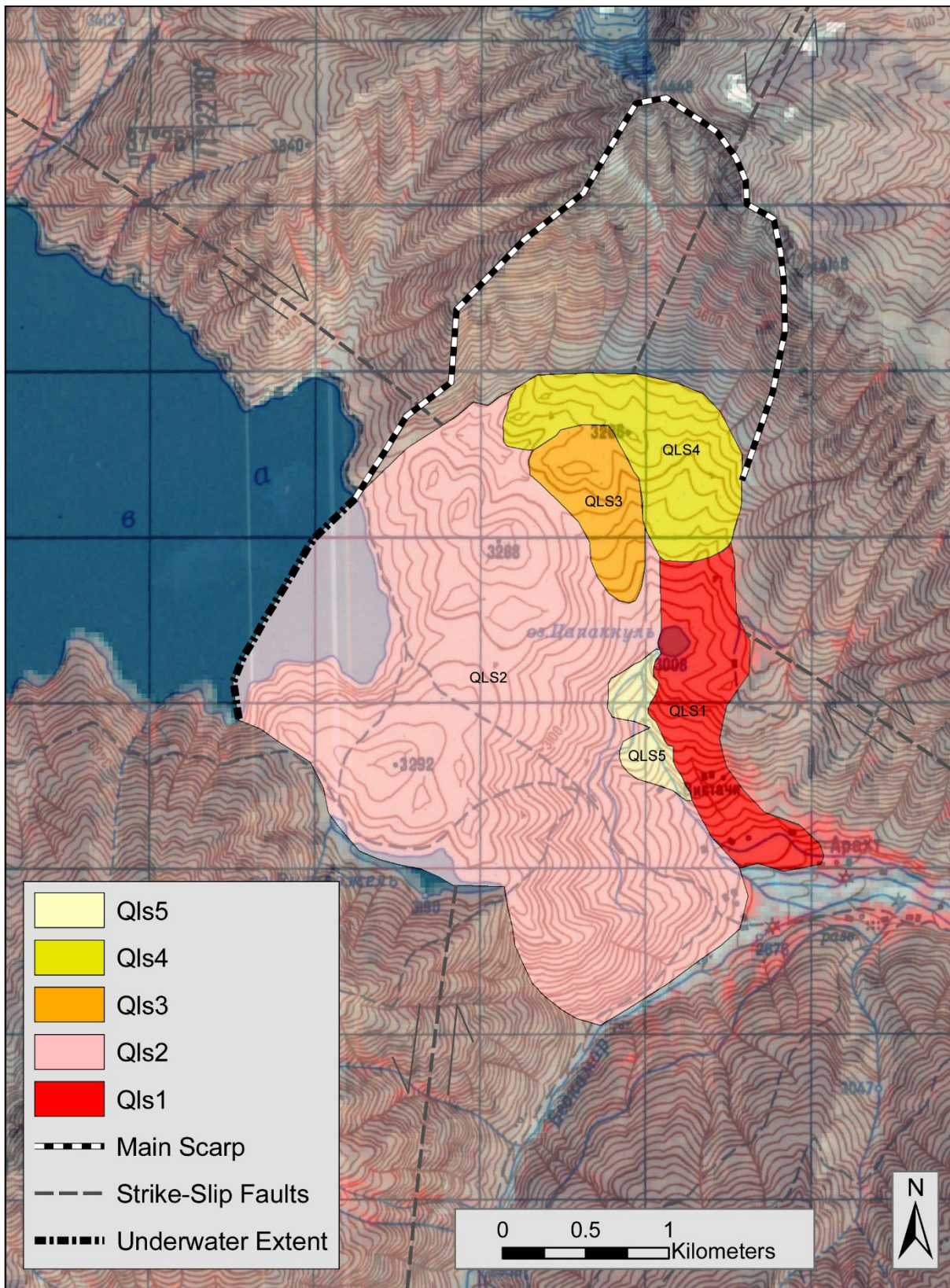
Шакли 4-6: Нақшаи банди чаҳили Шево, ки дар он минтақа ба ҳазорон сол қабл ташкил шудааст, шояд тавассути zilzila, ки боиси strike – slip fault шуда ва боиси фурӯ рафтани замин гардидааст. Лағзиши замин Q1s1 ва Q1s2 ҷойгоҳи фурӯрафтагии нишеби аввалӣ рух додааст, ки ба таъкиби он q1s3 ва каме дертар q1s4 воқеъ шуд. Чаҳил, ки дар чапи он қарор дорад, тавассути дарё пур шуд, ки аз тарафи чап ҷараёни (ғарб) ҷараён дорад ва баъдан дар тарафи рост(шарқ) ба Панҷ мерезад, ки дар якчанд килуметрӣ дуртар аз чаҳил ҷараён дорад.
