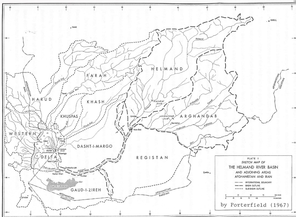
Шакли 4-7 А: Баъзе чахилҳои Афғонистон баъд аз он ки барфи зимистон об шуда пур мешавад ва баъдан дар тобистон гарм ва бо боди шадид хушк мешавад(боди 120 рӯза) .
