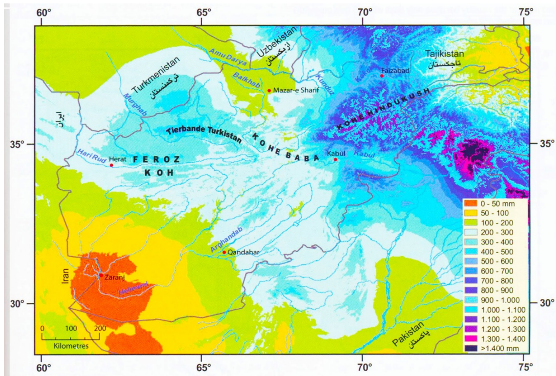
Шакли 5.2: Борандагии муттавасити солона дар Афғонистон ва кишварҳои ҳамҷавор ба
