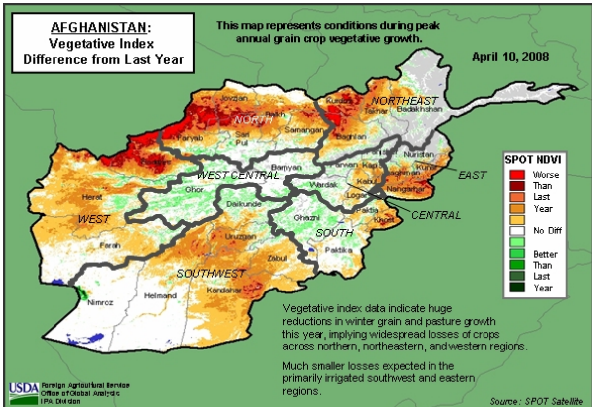
Шакли 5.7: Нақшаи Афғонистон дар соли 2008 индекси сабзичотро нишон медиҳад, ки аз тасвири қамари маснуъӣ сохта шудааст. Агар онро ба ба соли 2007 муқоиса кунед, дар қучо барои зироат харобтарин проблем вучуд дорад?
