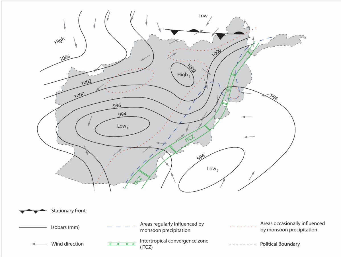
Шакли 5.6: Нақшаи оби Афғонистон дар тобистон мавқеияти муттавасити фишори пойин (ITCZ)- ро нишон медиҳад. Вақте ки борандагии мунсун ба Афғонистон ворид шавад, кадом ду мавзӯ рух медиҳад?
