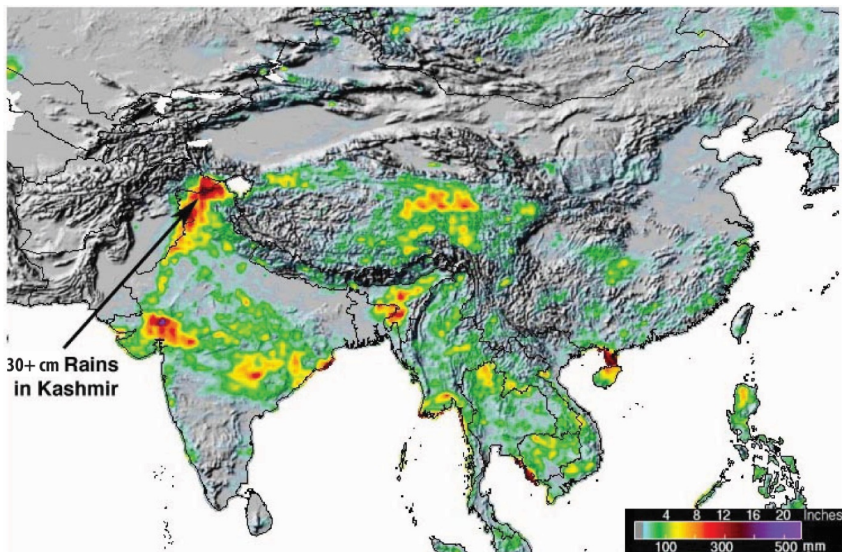
Шакли 5.4: Андозагирии борандагӣ TR ММ нишон медиҳад, ки сељоб да кучо рух медиҳад. Ин тасвир нишон медиҳад, ки дар септември 2014 356 миллиметр борон дар имтидоди сарҳадоти Ҳинд-Покистон, ки дар Кашмир борид, боиси сељобҳои азим шуданд. Ин борандагӣ натиҷаи фишори пойин, мунсуни қумӣ дар минтақа буд. Айни мавзӯ дар Афғонистон рух дод. Борандагии зиёд дар кучо аст?
